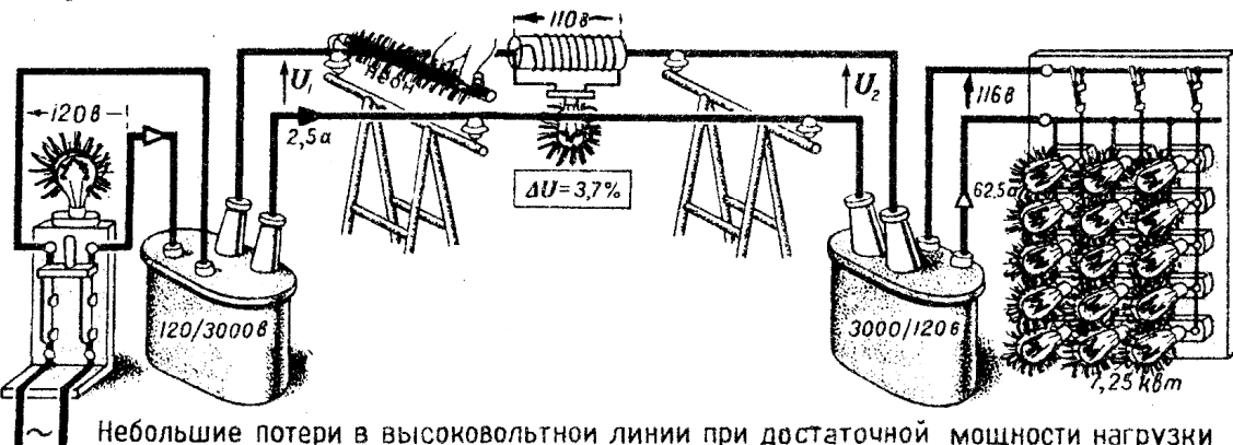
Ничтожные потери в высоковольтной линии при более мощном потребителе
