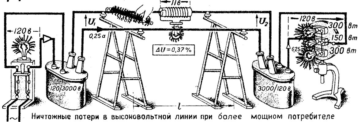
Значительные потери в низковольтной линии при более мощном потребителе
